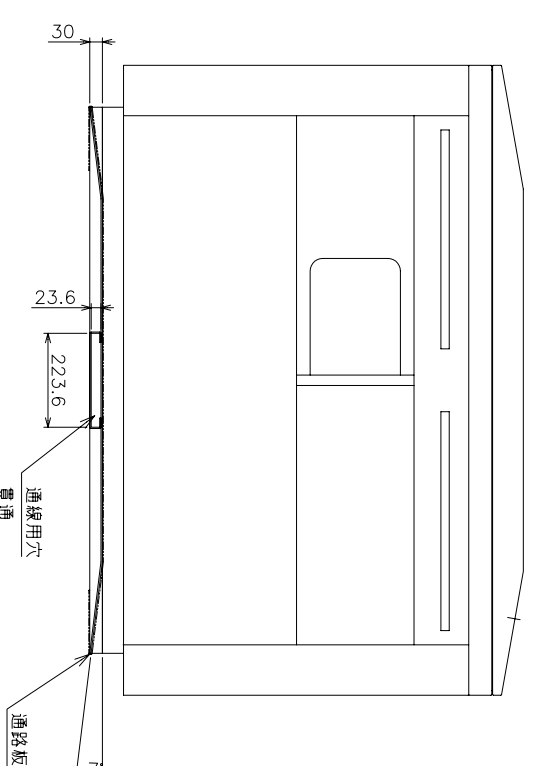
B 矢視図
